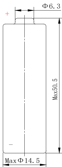
Dimensions in mm (GB1804-m)
